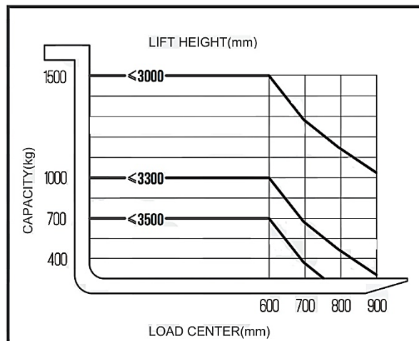
Рисунок 2. Графики грузоподъемности.
