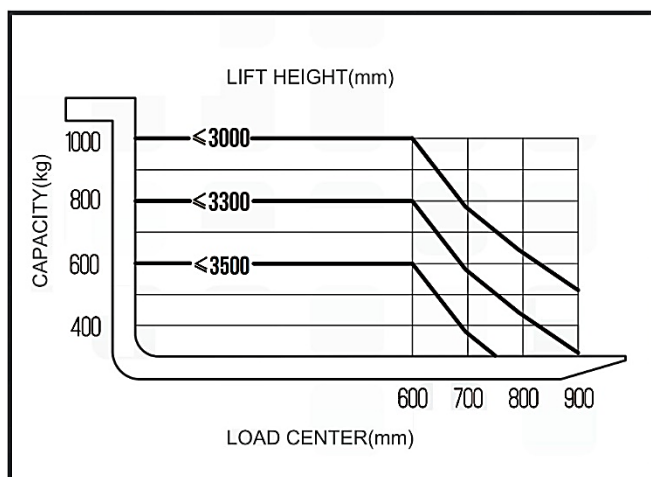
Рисунок 2. Графики грузоподъемности.
