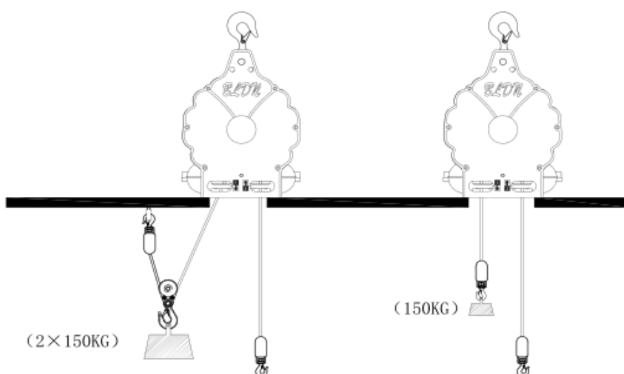
Схема использования функции двойной грузоподъемности
